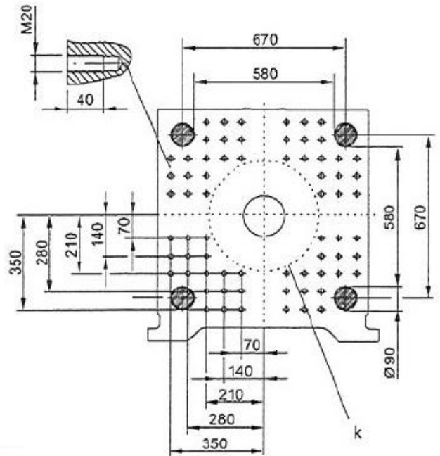
A - A
