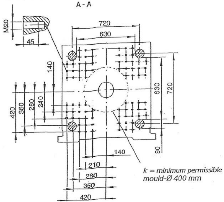
Fixed platen
