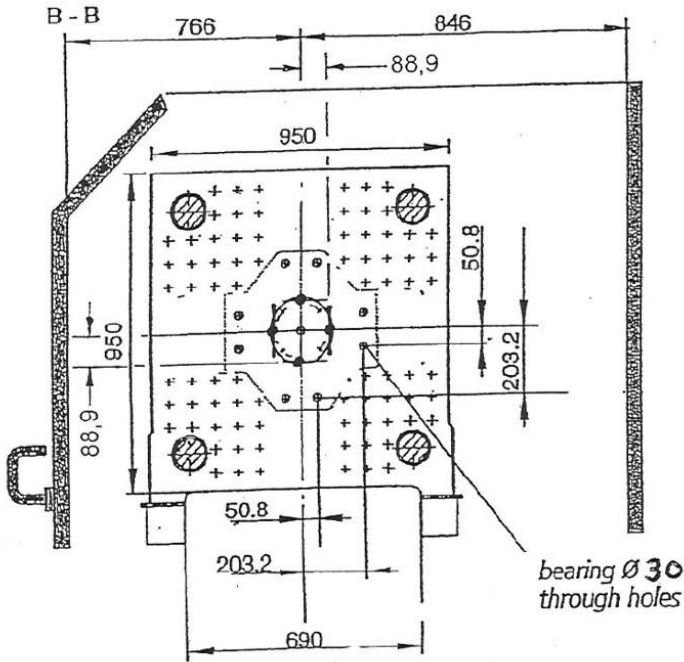
Moving platen
